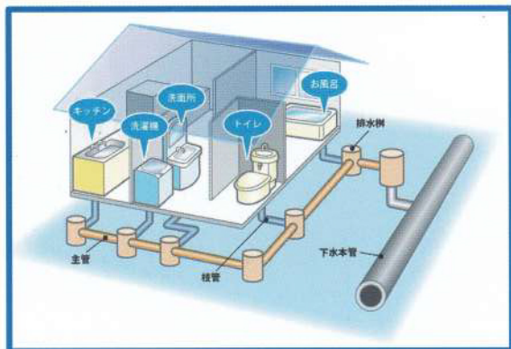
家庭の排水桝の仕組み
